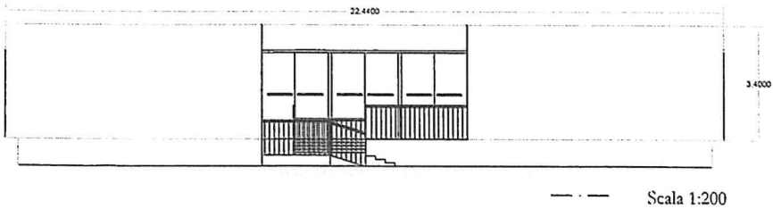
PROSPETTO FRONTALE
